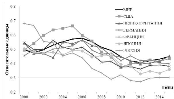
Рис. 7. Концентрация в подобластях (индекс Херфиндаля – Хиршмана): группа G 1 (жирная линия соответствует концентрации мирового «портфеля»)
