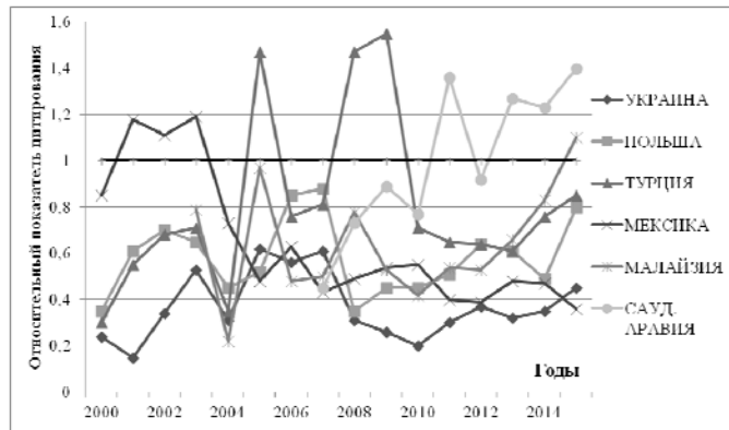
Рис. ПЗ.3. Национальный импакт У-нано статей относительно среднемирового уровня: группа G_5
