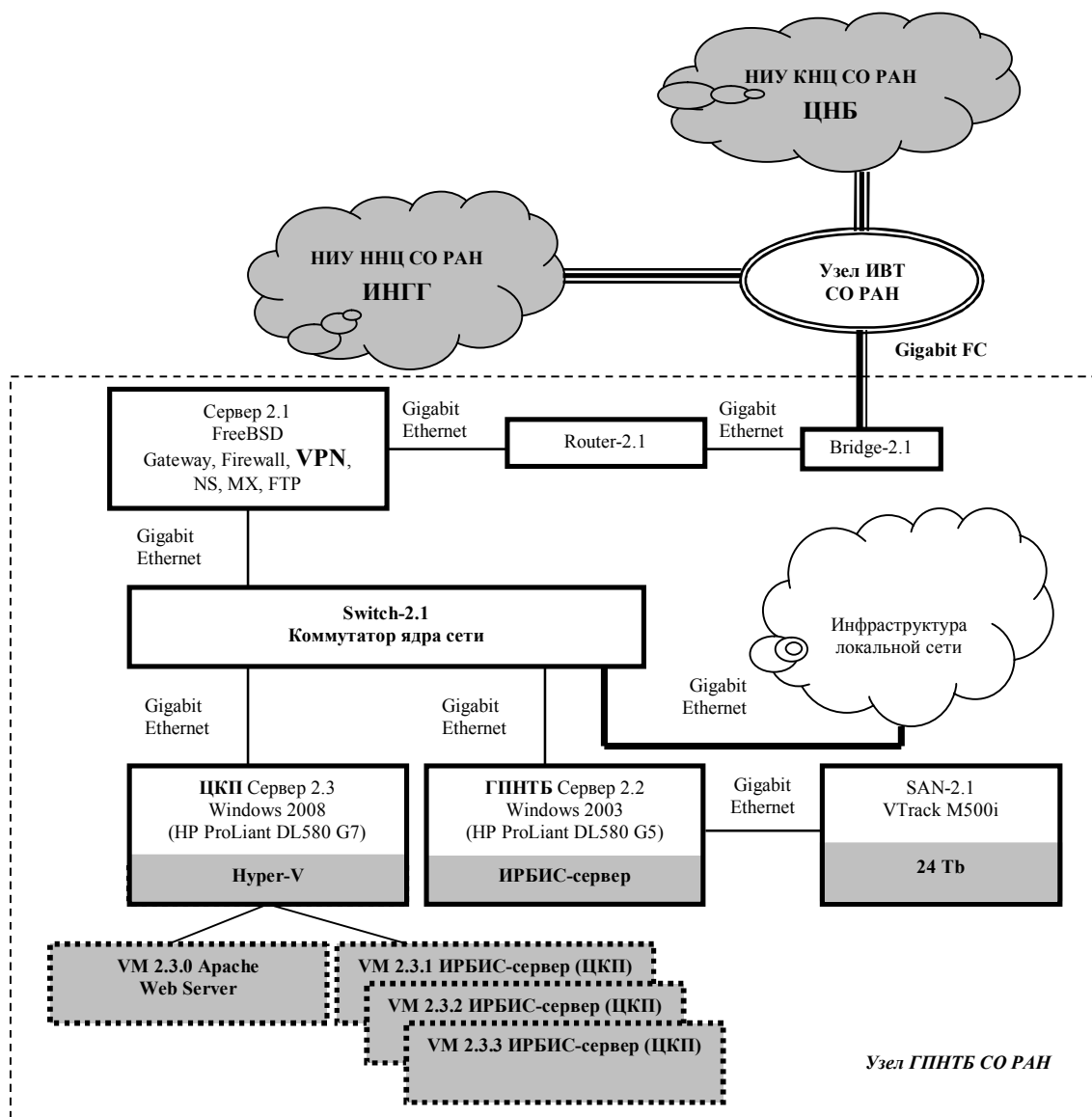
Рис. 1. Блок-схема серверного узла ГПНТЬ СО РАН в общей схеме коммуникаций
